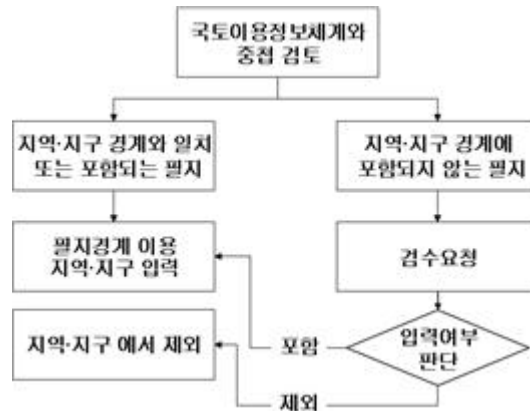
[그림 3] 지적기준 도형자료의 입력 절차
